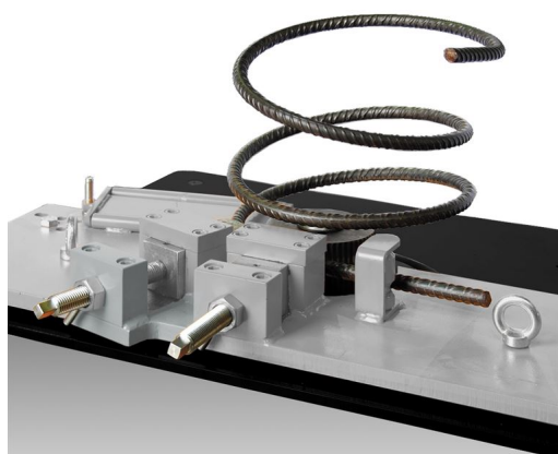
Spiralni uređaj S/18 TECMOR za P30-S, P36-S, PGT32/25
